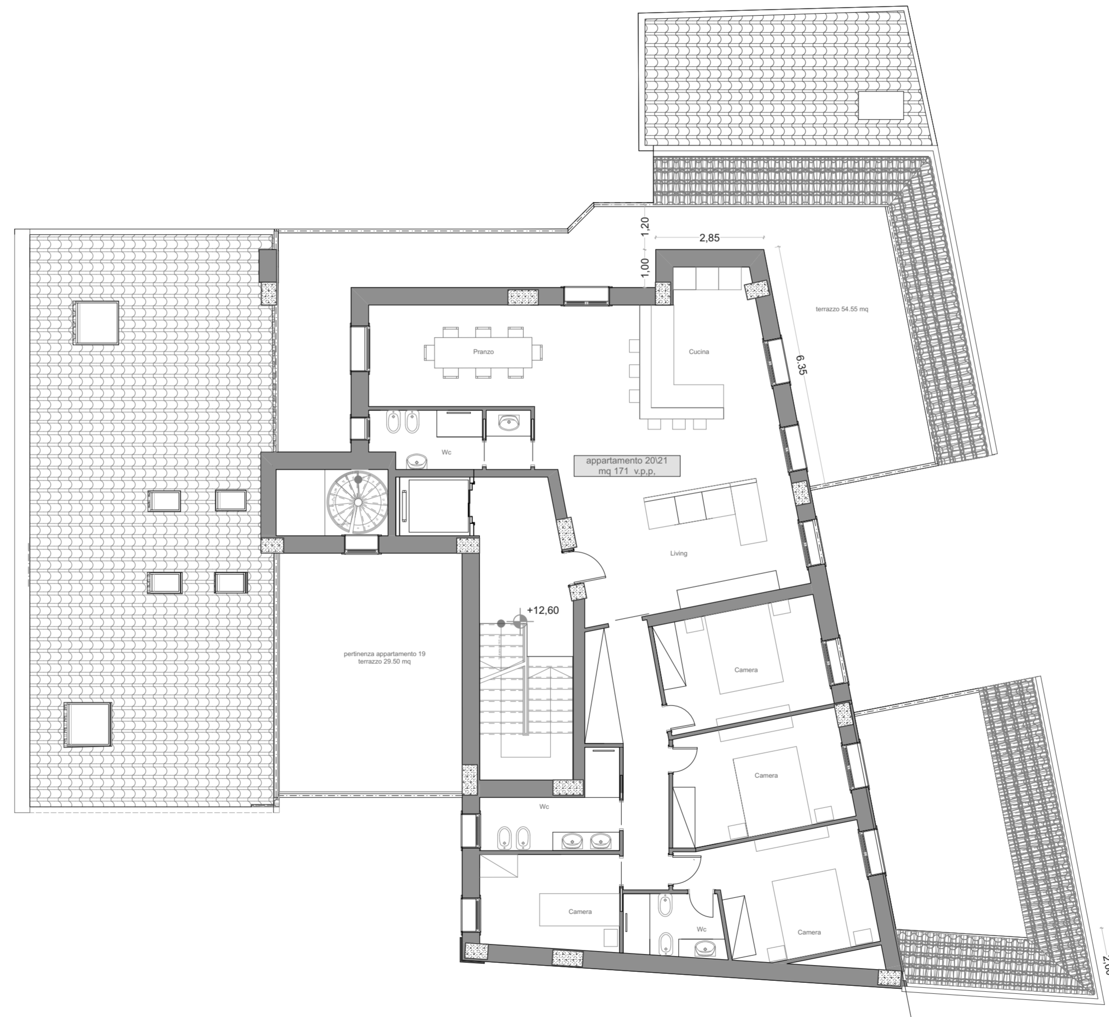
Pianta 4°livello - Unico Attico
